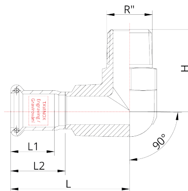
Technický náčrt
