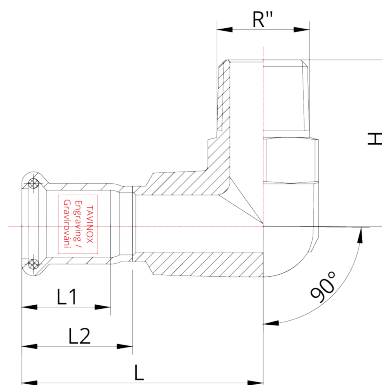
Technický náčrt
