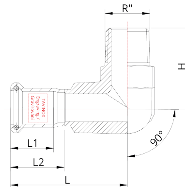
Technický náčrtek
