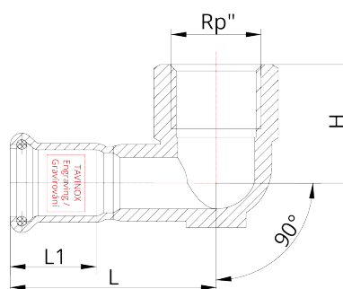
Technický náčres
