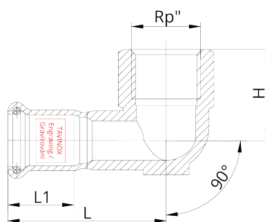
Technický náčrt
