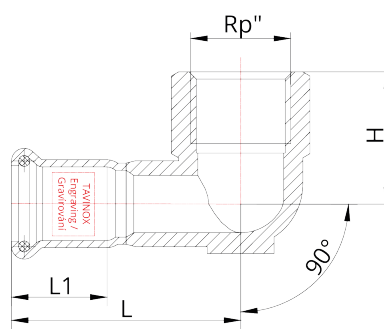
Technický náčres
