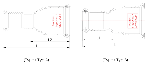
Technický nákres
