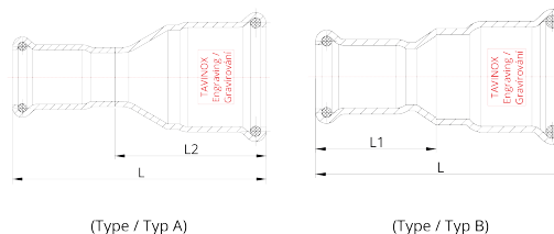
Technický nákres
