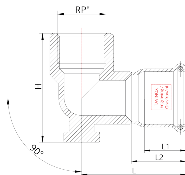
Technický náčrtek
