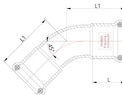
Technický nákres
