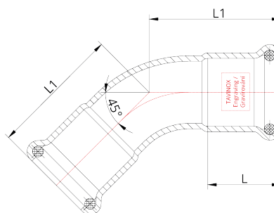
Technický náčrt
