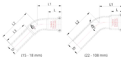
Technický náčrt
