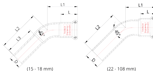
Technický náčrt
