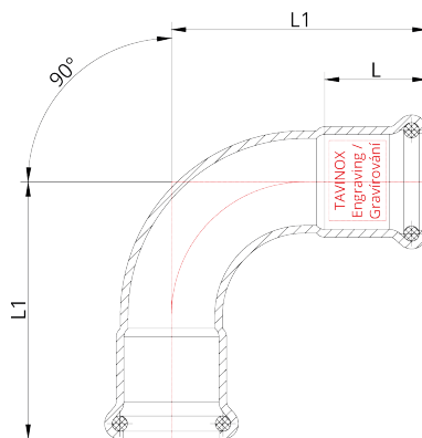
Technický nákres
