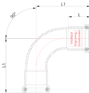
Technický nákres
