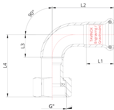
Technický nákres
