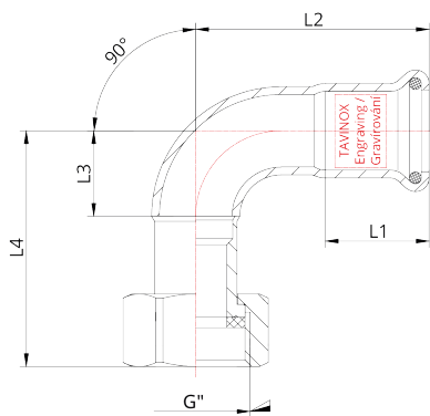
Technický nákres
