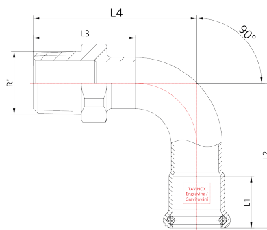
Technický náčres
