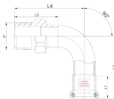
Technický náčrt
