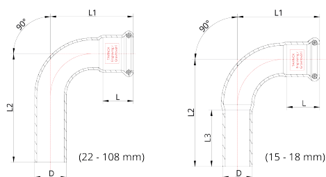
Technický náčrt
