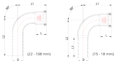
Technický náčrt
