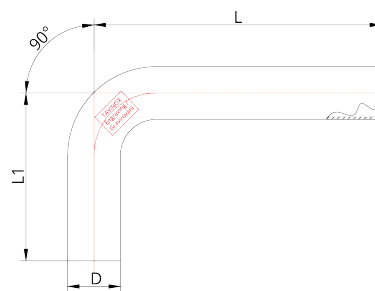
Technický nákres
