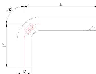
Technický nákres
