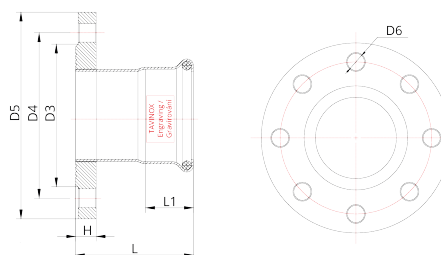
Technický náčrtek
