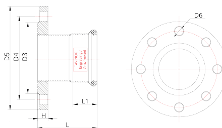
Technický nákres
