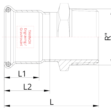
Technický náčres
