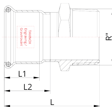
Technický nákres
