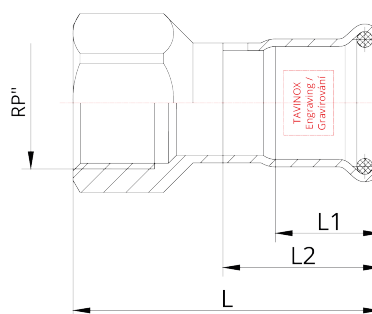
Technický nákres
