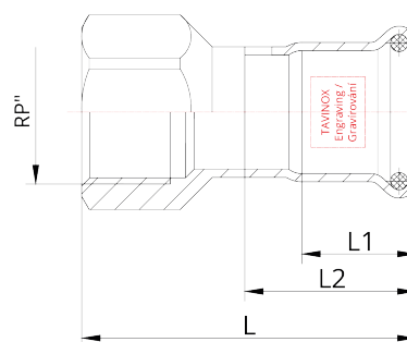
Technický nákres
