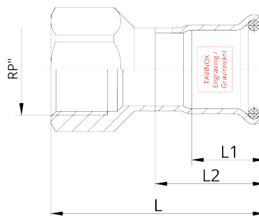
Technický nákres
