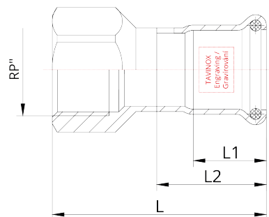
Technický nákres
