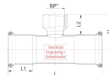
Technický náčres
