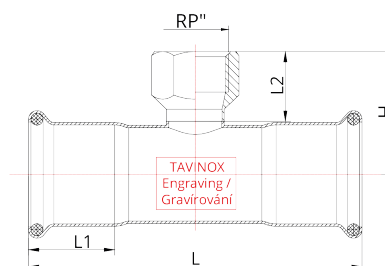
Technický náčres
