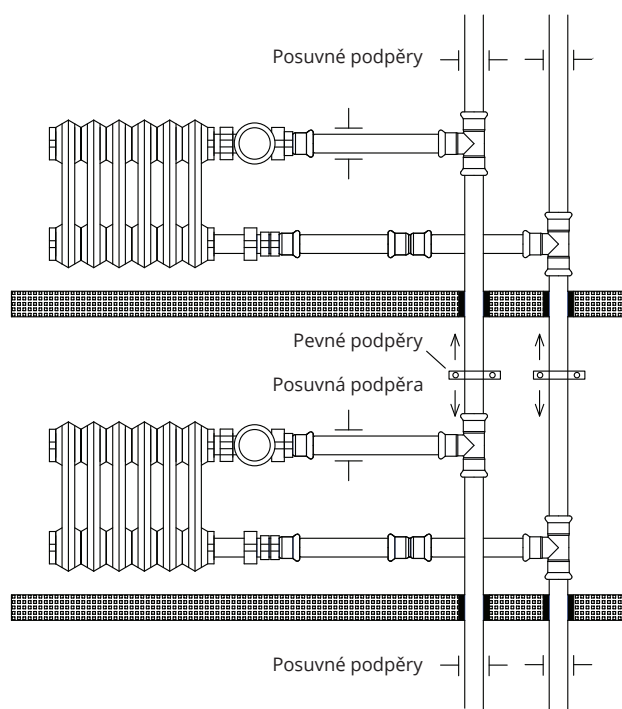
Příklad správného upevnění dlouhých úseků
